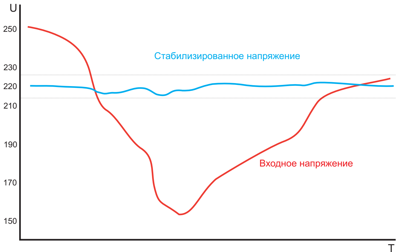
Электродинамический принцип регулирования напряжения.
